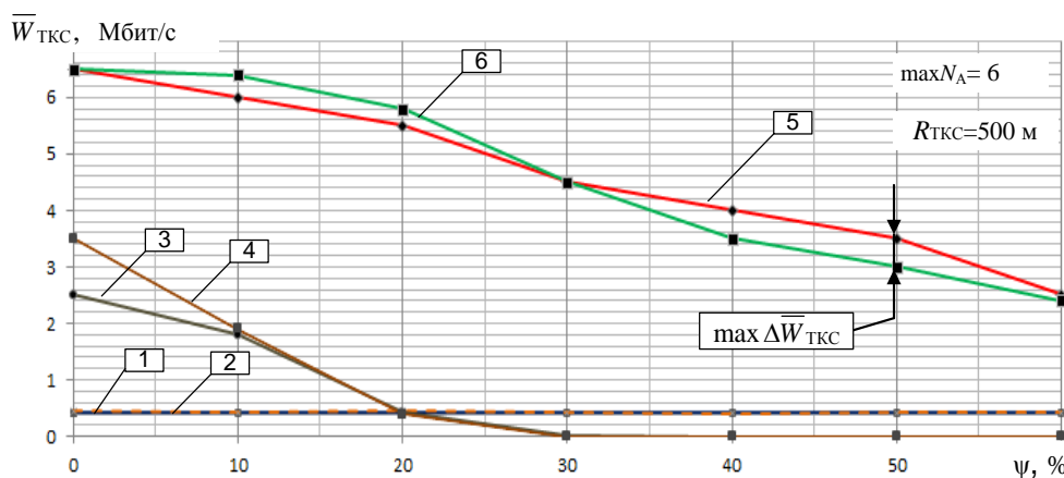
Рис. 7. Зависимости средней пропускной способности ТКС СН от степени воздействия ВДФ для различных типов структур при N_{a6} = 6 и R_{ТКС СН} = 500 м
