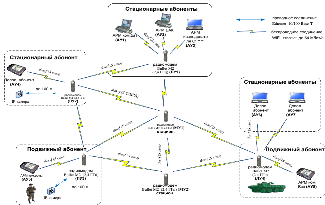
Рис. 6. Состав экспериментального макета сегмента ТКС СН
