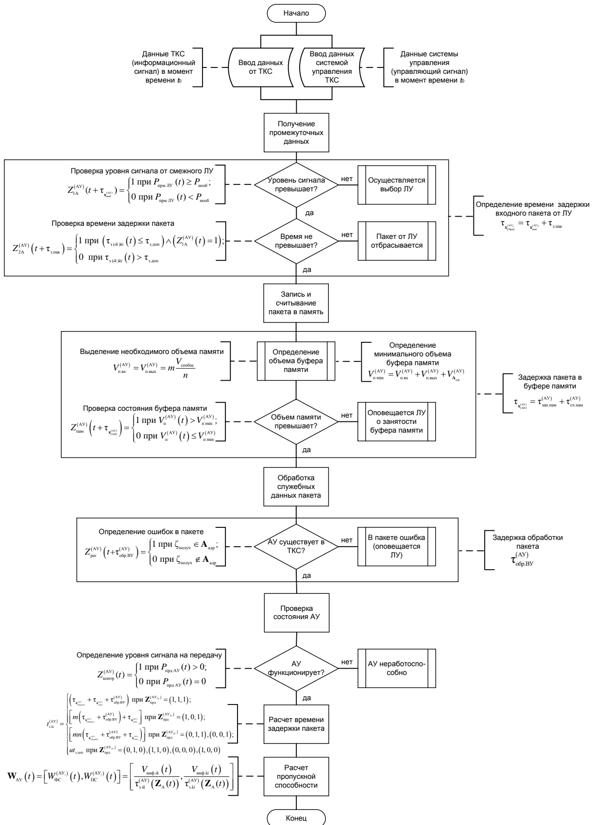
Рис. 2. Схема процесса определения пропускной способности AY при обработке пакетов сообщений
