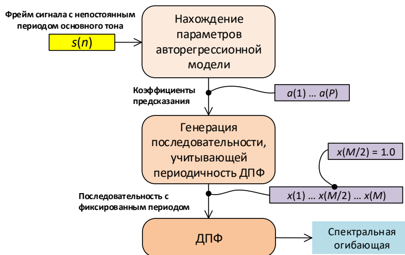
Рис. 1. Схема вычисления спектральной огибающей
