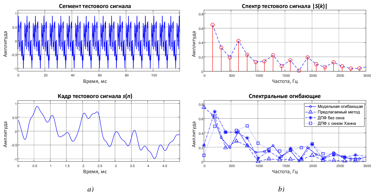
Рис. 2. Тестовый сигнал (а) и соответствующие спектральные огибающие для одного кадра (б)
