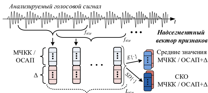
Рис. 4. Принципы формирования надсегментных признаков
