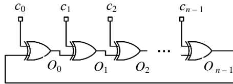
Рис. 4. Управляемый кольцевой осциллятор Fig. 4. Controlled ring oscillator
